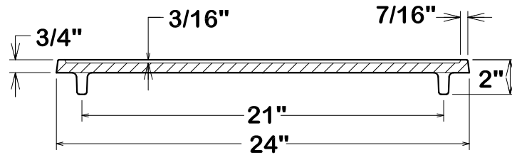
VIEW A-A
